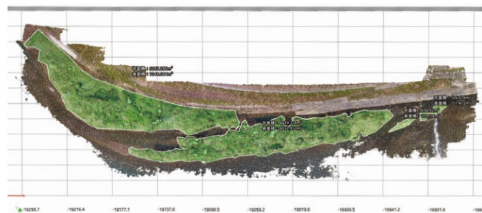
ドローンで地形を空撮し、コンピュータを用いて3次元処理解析をしたもの
